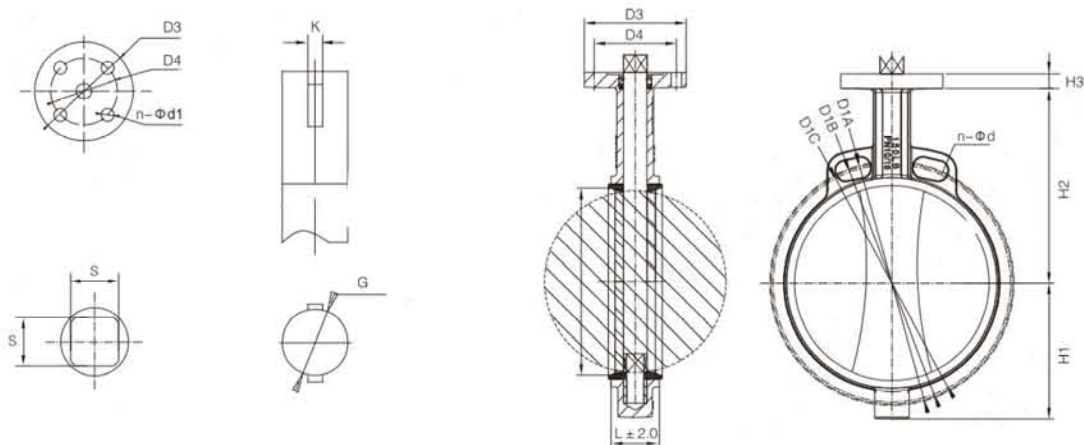
PN10&PN16&150LB
